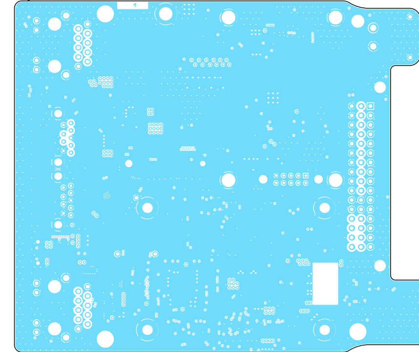
Layer 4 (Scale 1:1)
