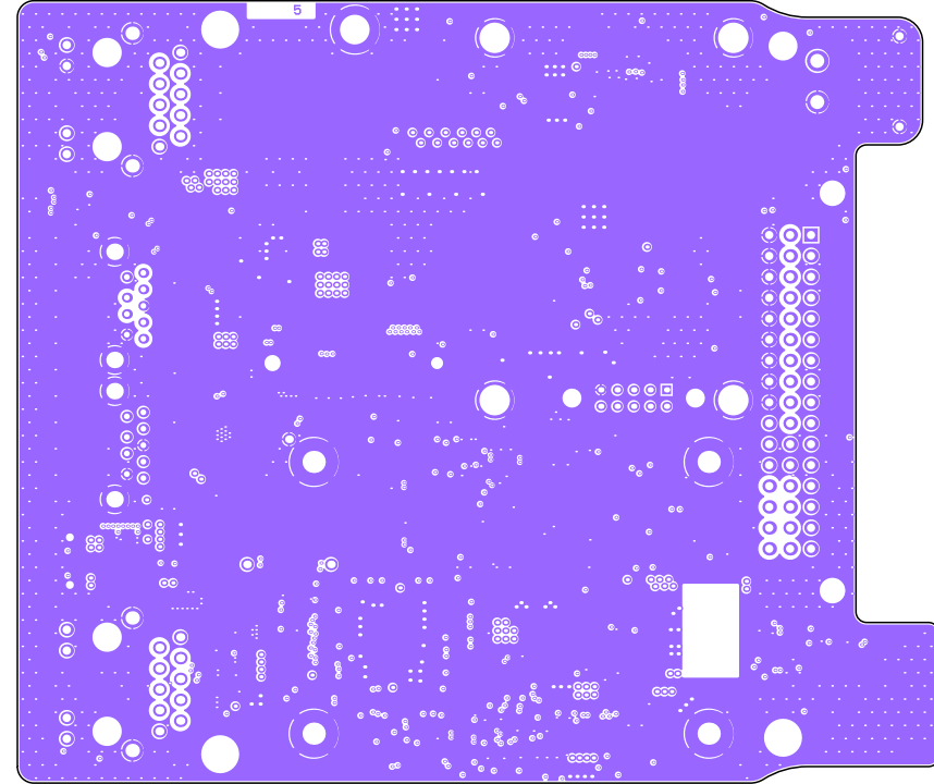
Layer 5 (Scale 1:1)
