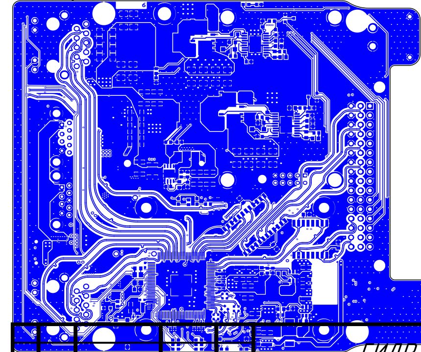
Bottom Layer 6 (Scale 1:1)
