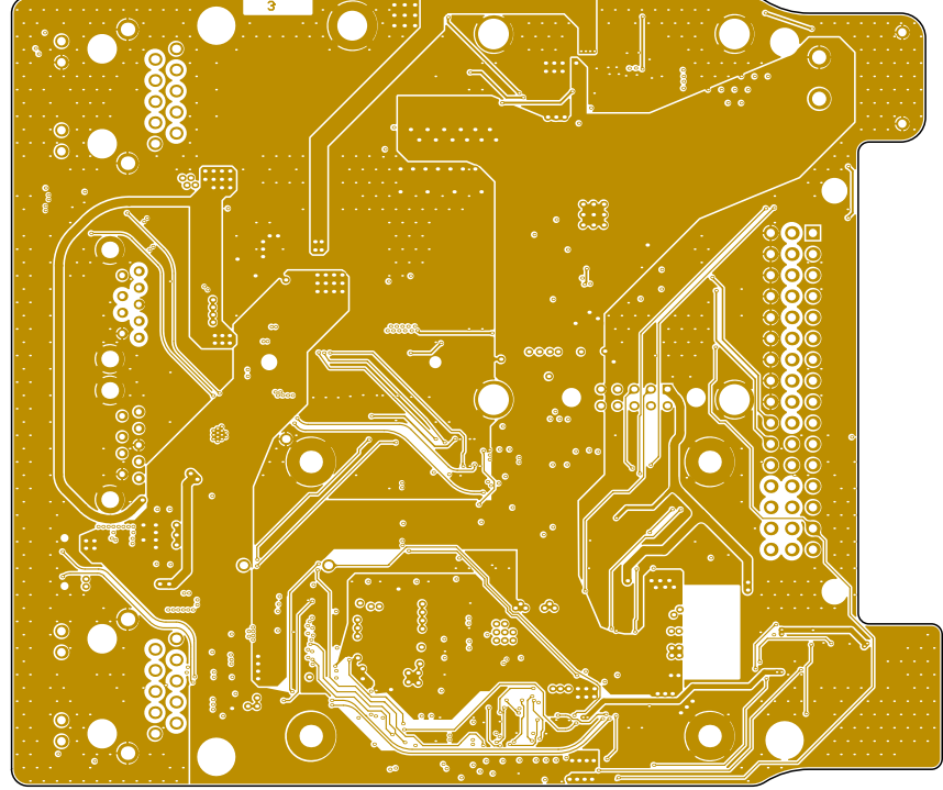
Layer 3 (Scale 1:1)
